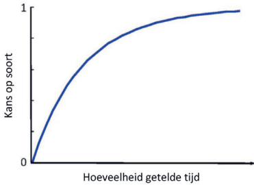
Figuur 2. Detectiecurve; naarmate er langer wordt geteld, neemt de kans om een soort waar te nemen ook toe. Bij lastige soorten is de curve minder steil dan bij gemakkelijke soorten.
